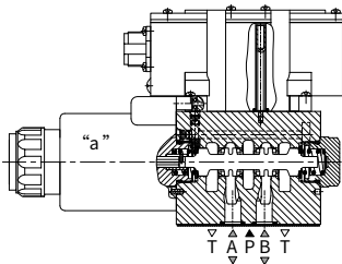
型号 4WRAE 10...A-L2X/...
